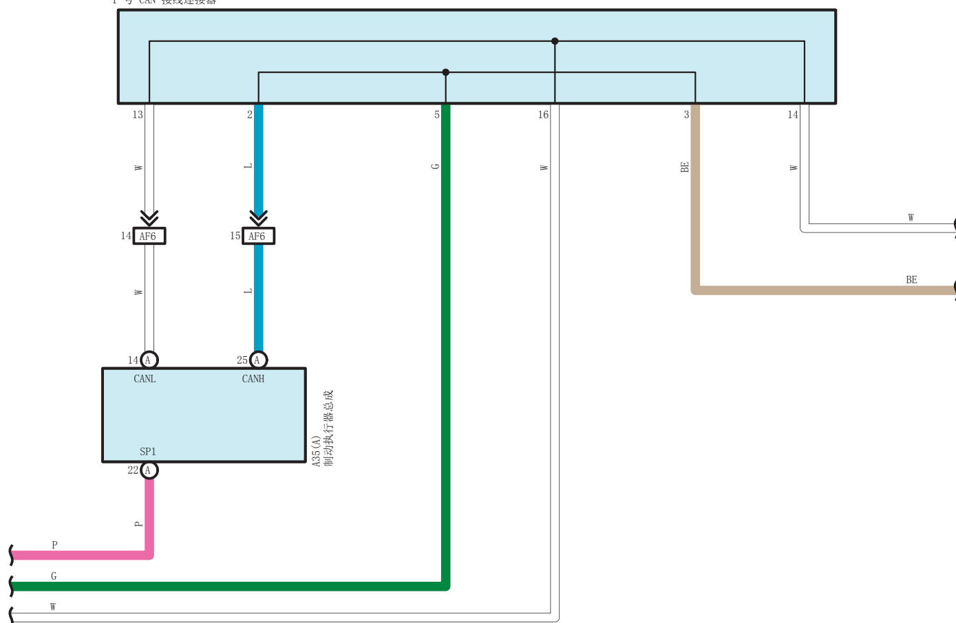
F62 1 号 CAN 接线连接器
