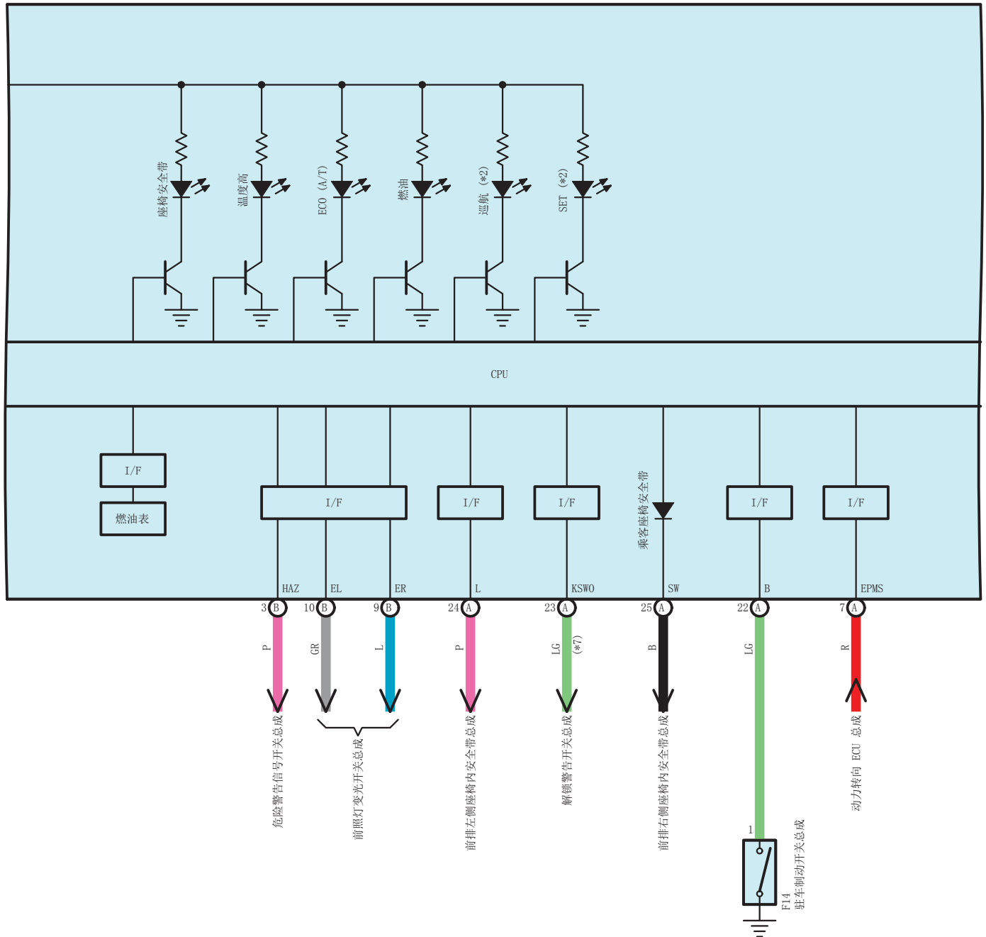
F38 (A), F39 (B) 组合仪表总成
