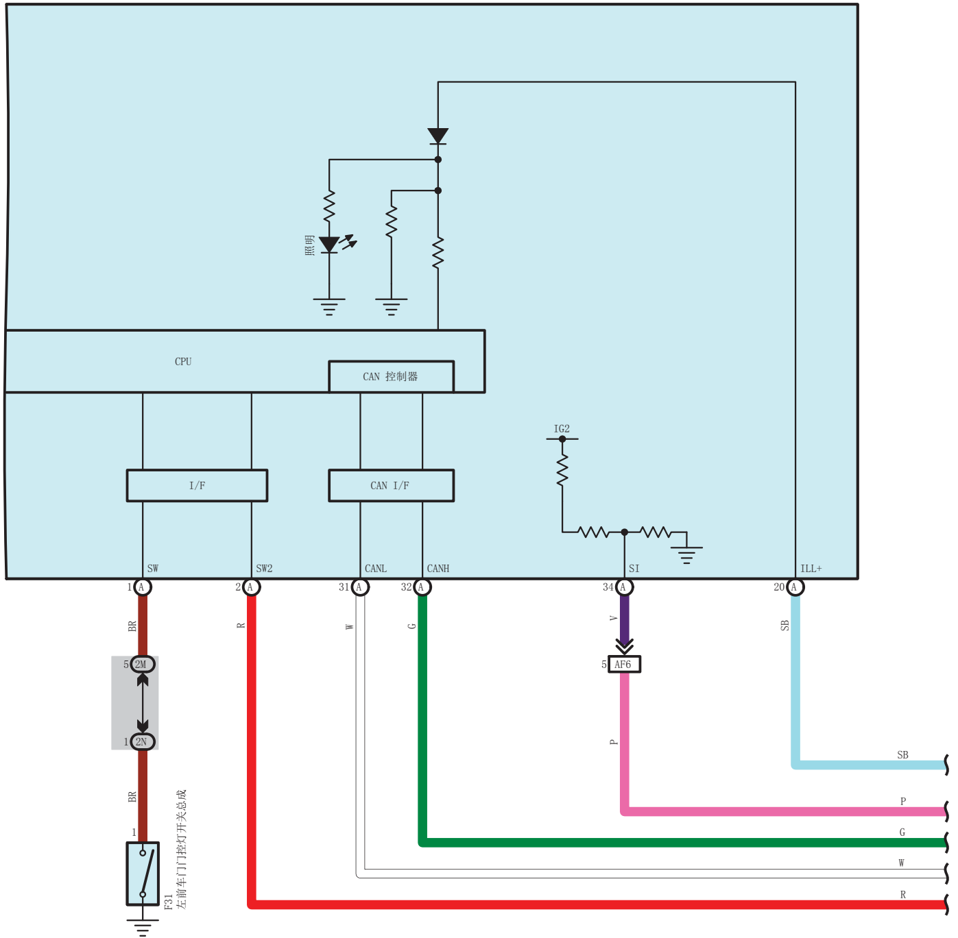
F38 (A), F39 (B) 组合仪表总成
